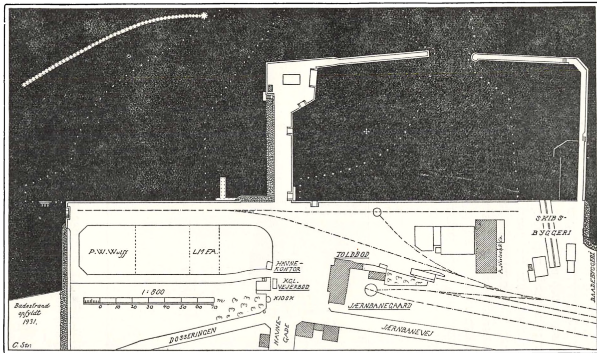
Fig. 11. Stubbekøbings tredje Havn efter 1911 samt den i 1931 byggede fjerde Havn Vest for. De Arealer i begge Bassiner, der ligger inden for de punkterede Linier, har en Vanddybde paa 6 m (Tegningen fra 1932).
