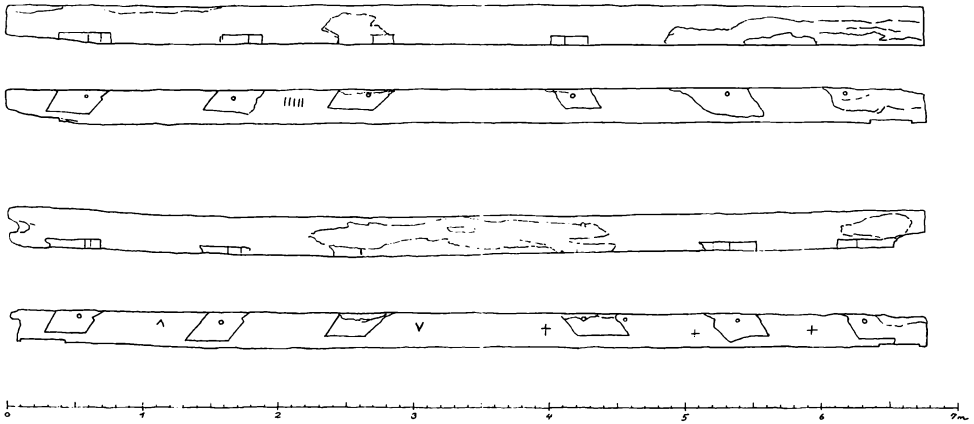
Opmåling af de to gavbjælker fra klokkestokværket, plan og opstalt.
