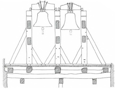
Opmåling af klokkestolens buk nr. II, opstalt af østtiden. Bukkens lighed med det græske bogstav pi, har givet konstruktionen navn.
