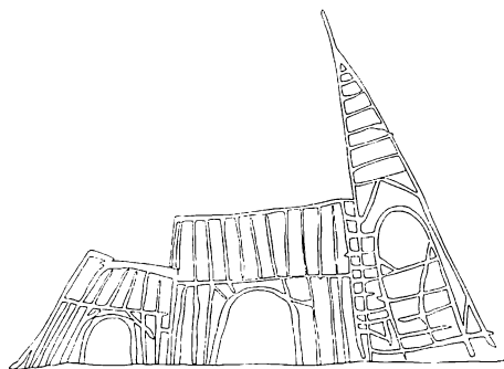
Tømrerens rids af en kirke (Hunseby): 2. spær i syd-siden over skibet.
