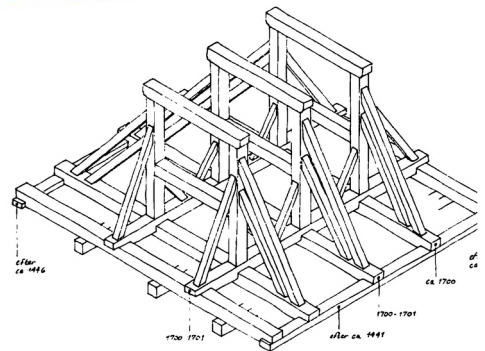
Isometri af klokkestolens tre bukke (nord opad til venstre). Årstallene angiver den dendrokronologiske datering af tømmeret.
