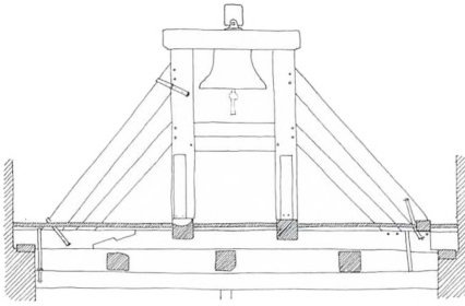
Opmåling af klokkestolens sydside. De to yderste bjælker, der er snittet igennem, viste sig at stamme fra den ældre klokkestol.
