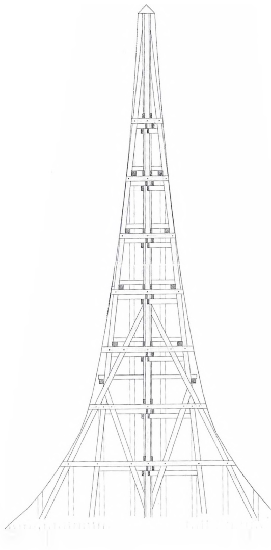
Et af tre snit i det ottende projekt til spiret i Fuglse.
