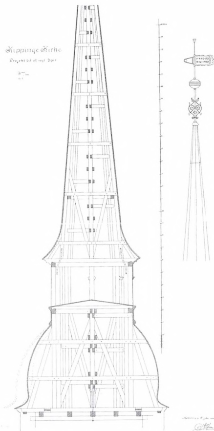
Projekt til nyt spir på Kippinge Kirke. Januar 1910.
