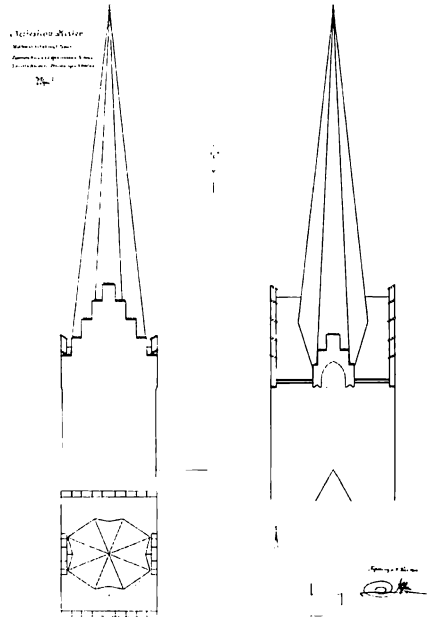
Skitseforslaget til det nye spir viser det gamle i profil, så ingen kan være i tvivl om det nye vil blive flottere og en pryd for byen. Tegning nr. 1. 1. februar 1904.
