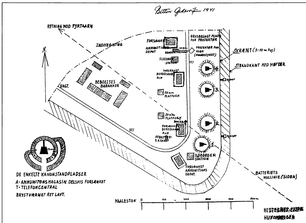
Kaptajnløjtnant Marckmanns skitse af kanonbatteriet på Gedser Odde. Rigsarkivet.
